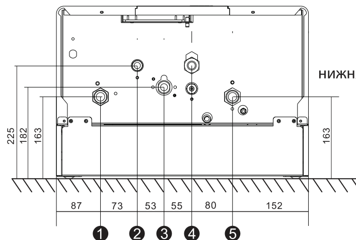
Рис. 2. Габаритные и присоединительные размеры. Двухконтурные модификации.
