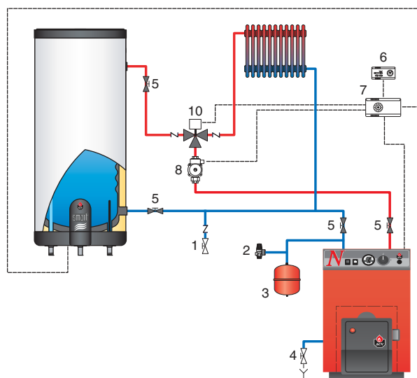
Бойлер с 3x-ходовым моторизированным клапаном. Вариант вертикального монтажа.
