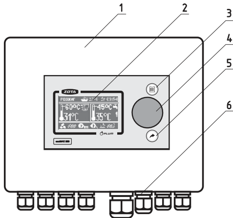
Рис. 5 Пульт управления
