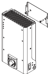
Рисунок 10а. Крепление стабилизаторов Штиль IS350 и IS550 на ровной вертикальной поверхности
