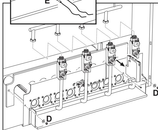
мал. 7 - Демонтаж та очищення вузлу палиників
