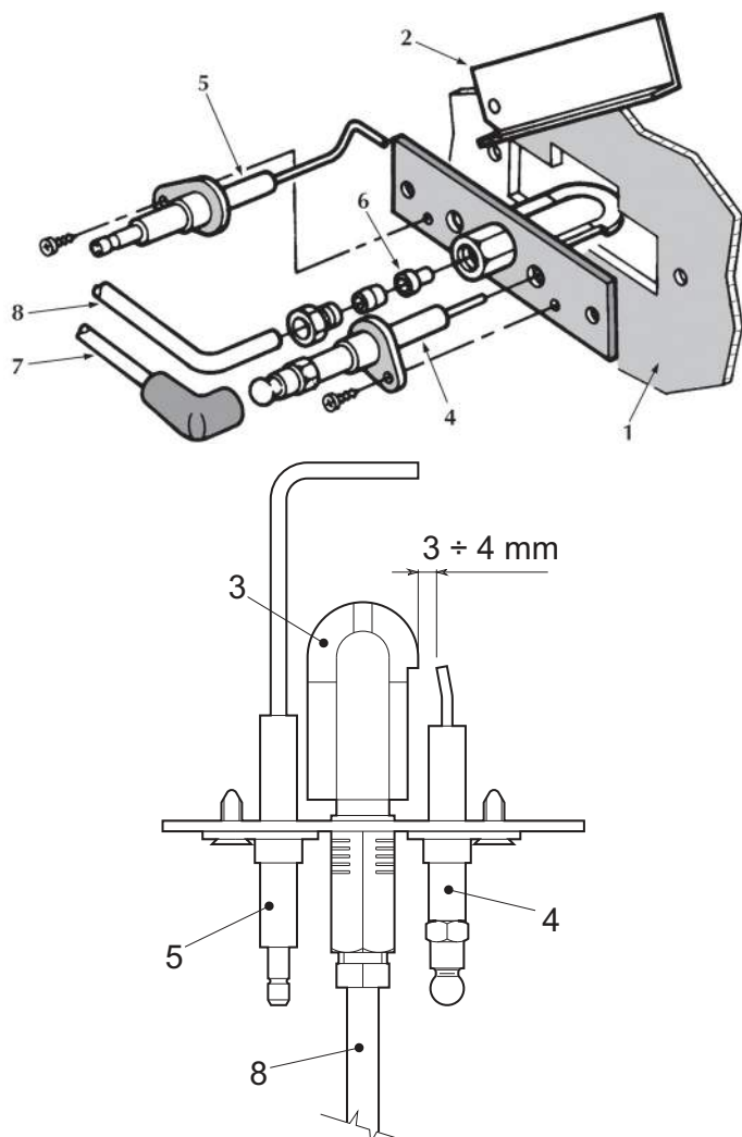
fig. 8 - Brûleur pilote
