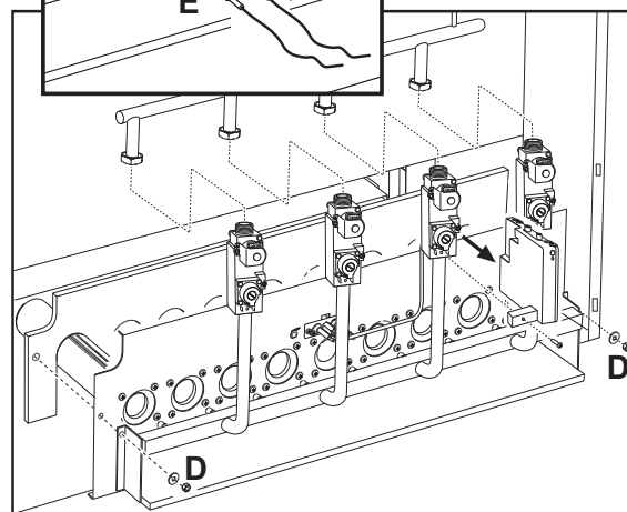
fig. 7 - Démontage et nettoyage des brûleurs
