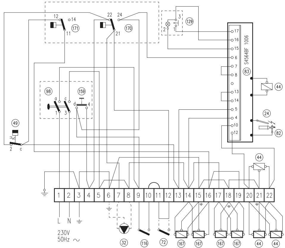
şek. 14 - Elektrik bağlantı şeması, mod. 153 ÷ 289
