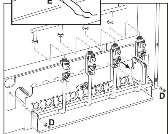
мал. 7 - Демонтаж та очищення вузлу пальників
