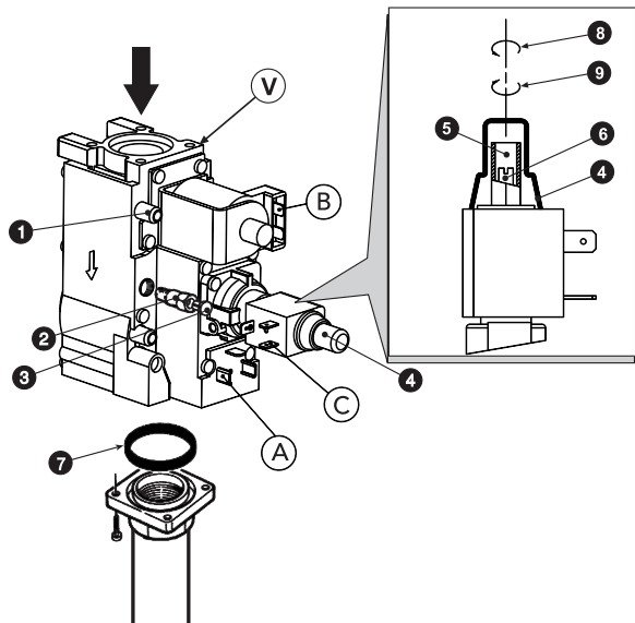
الشكل 4 - تبديل غاز التغذية التشغيلية
