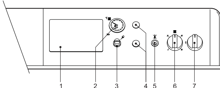
fig. 1 - Pannello comandi
