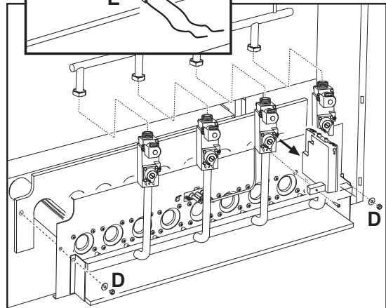
şek. 7 Brülörlerin sökülmesi ve temizlenmesi
