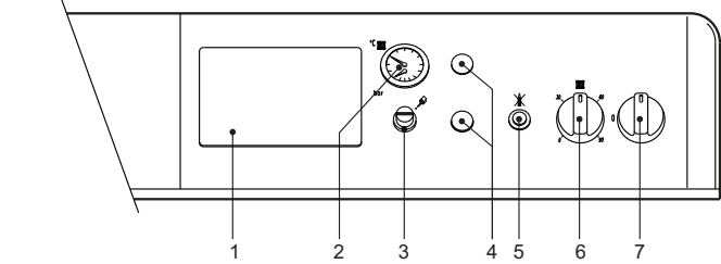
мал. 1 - Панель команд
