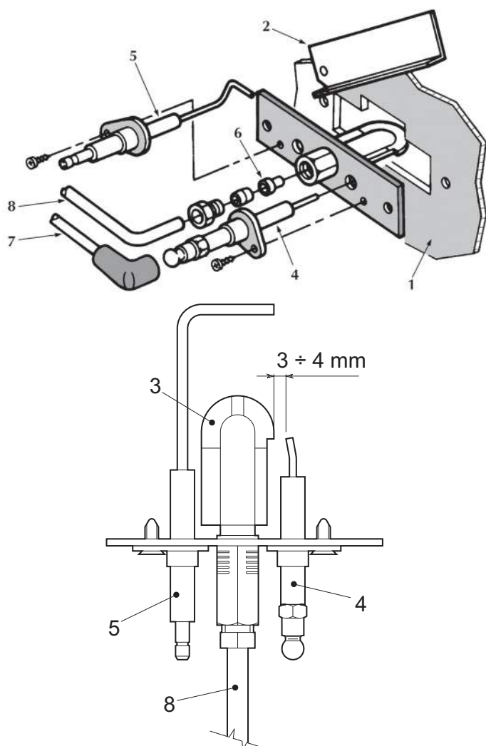
fig. 8 - Brûleur pilote
