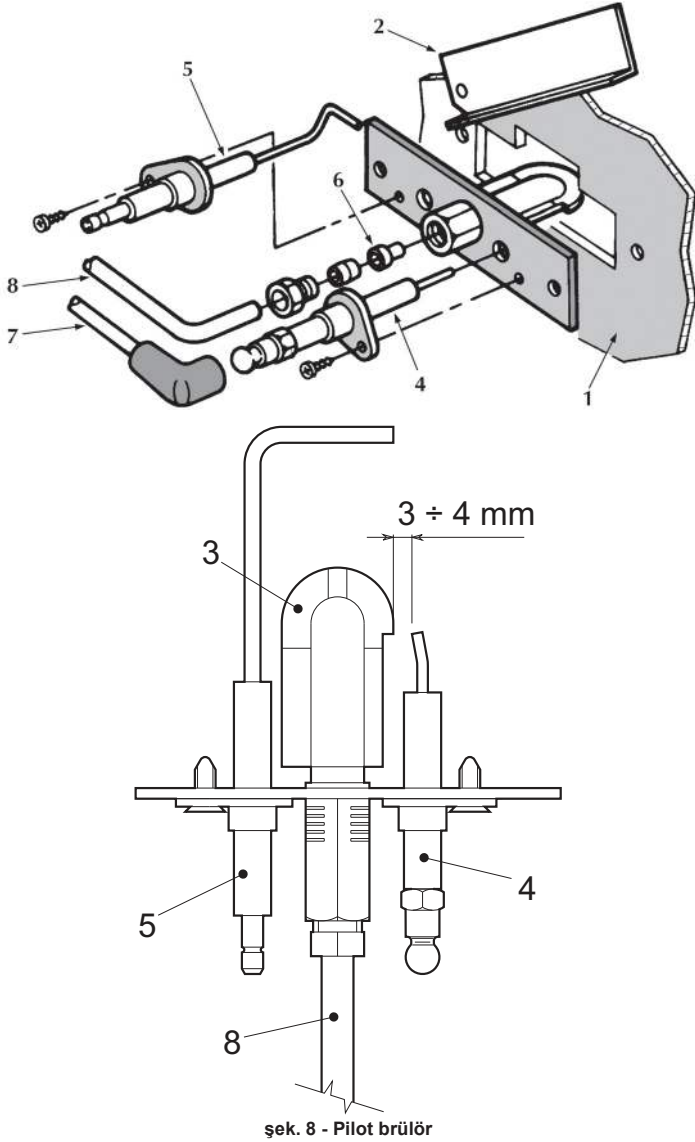
şek. 8 - Pilot brülör
