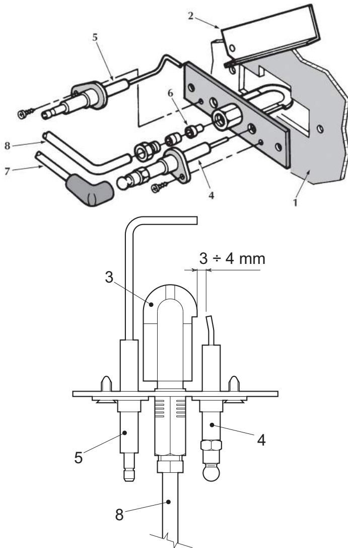
fig. 8 - Quemador piloto
