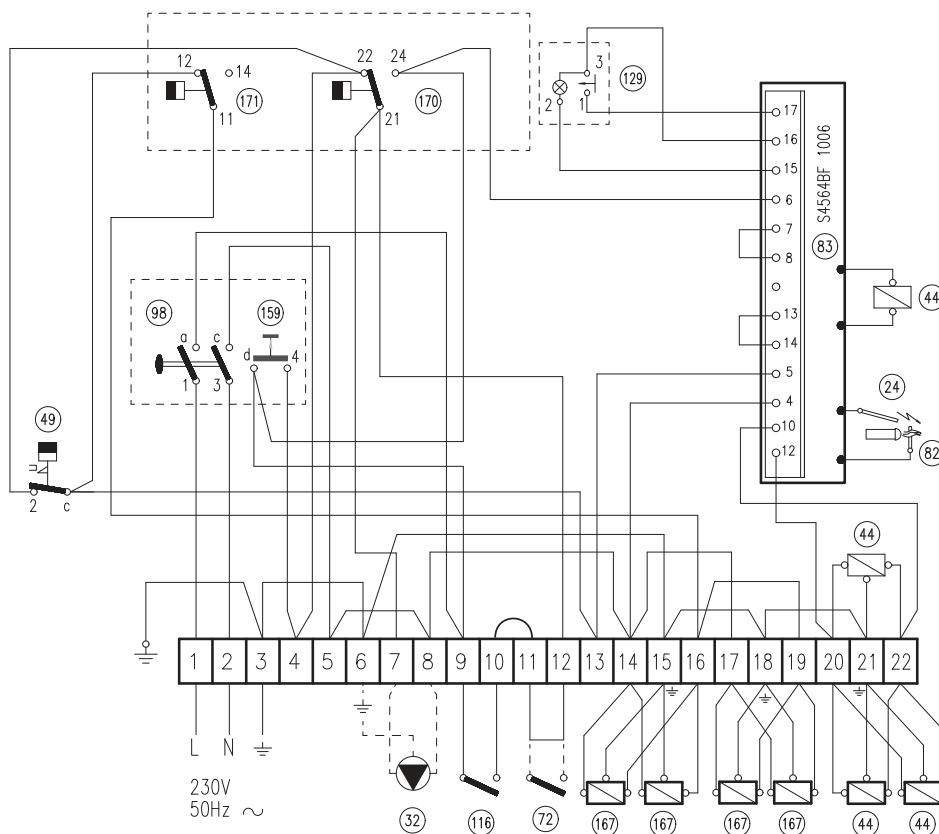
Schéma électrique de base mod. 153 ÷ 289
