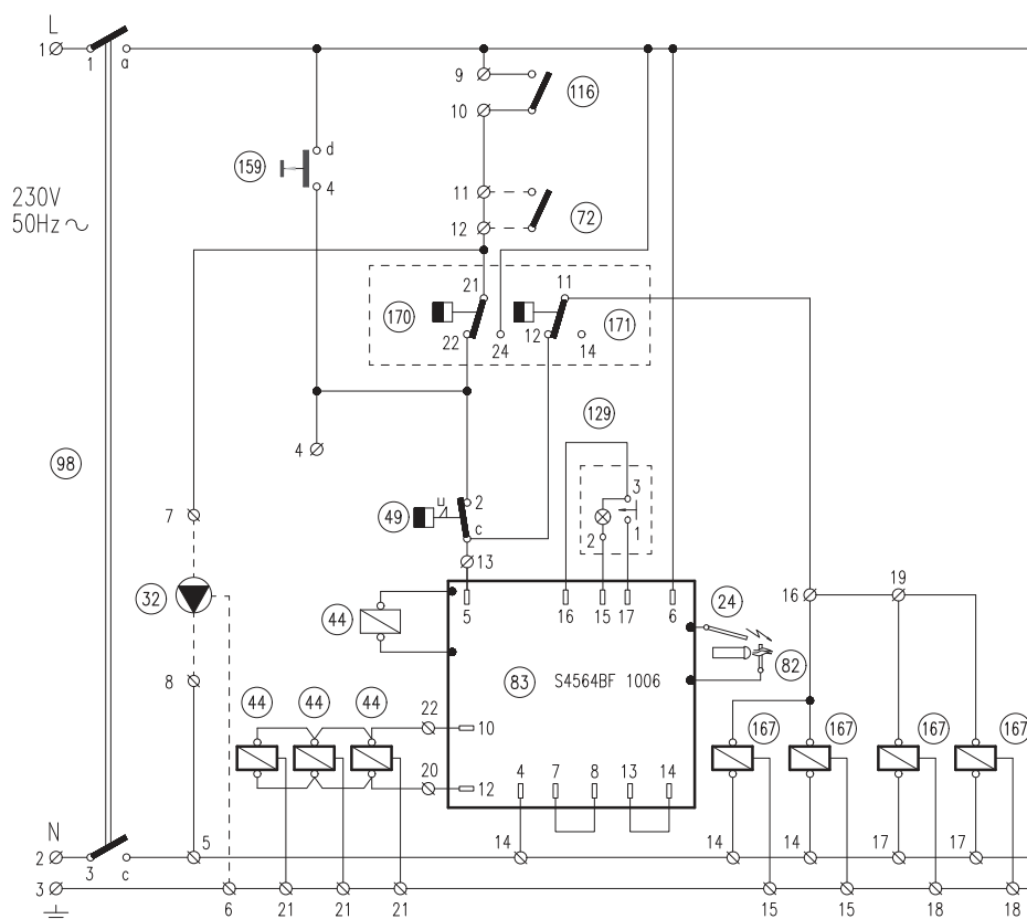
Schéma électrique de base mod. 153 ÷ 289
