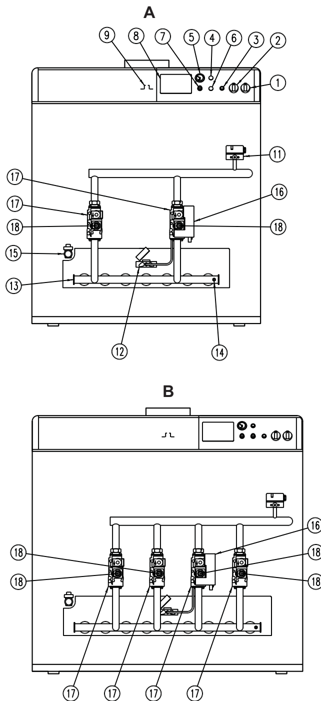
fig. 11 - Vista generale e componenti principali
