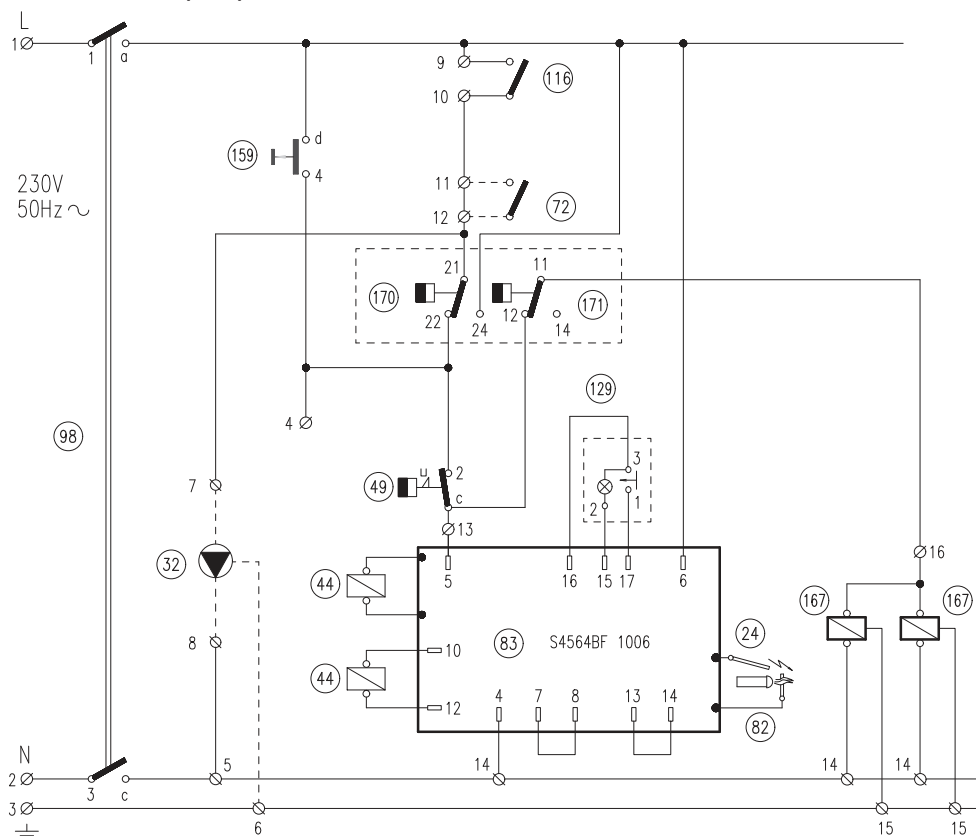
Schema elettrico di principio mod. 119 - 136
