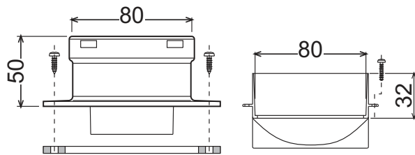
рис. 30 - Соединительный элемент для отдельных труб
