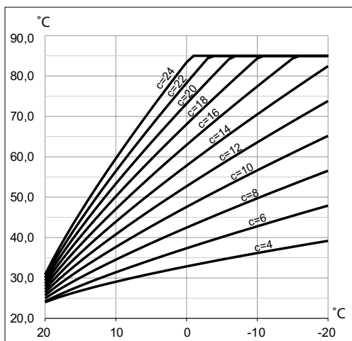
Коэффициент наклона кривой нагрева
