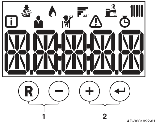
Рис.34 Панель управления
