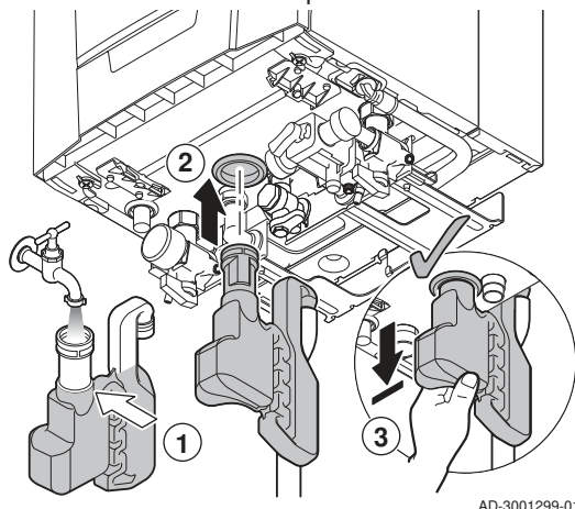
Рис.35 Заполнение сифона
