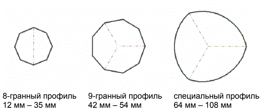
Схема 4: поперечный разрез пресс-соединений при помощи пресс-насадок и хомутов SANHA®
