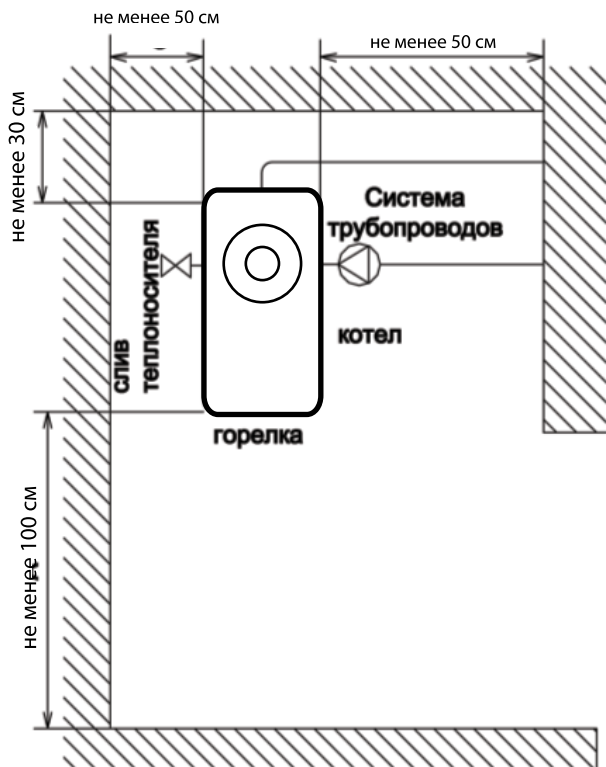
Рисунок 14. Установка котла
