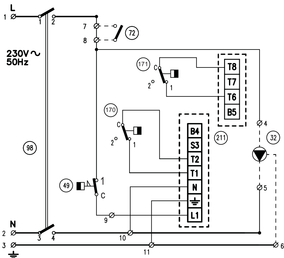
fig. 9 - Schéma électrique de base EL-DB N 95
